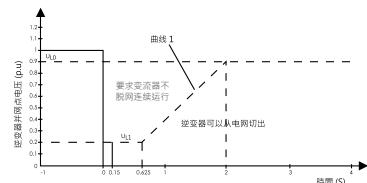
低电压穿越 (LVRT) 测试 NB/T 32004-2018
