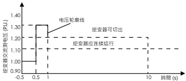
高电压穿越 (HVRT) 测试 NB/T 32004-2018
