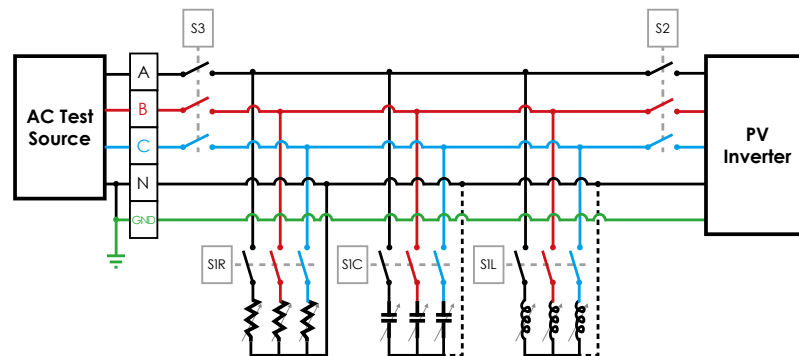
反孤岛测试配置图 (IEEE1547.1-2020)
